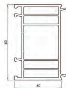
COMPENSATORE 50 MM - 68056
