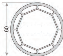
CONNETTORE TUBOLARE - 57061
