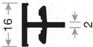
CONNETTORE H - 57052
