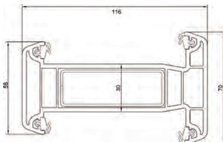
CONNETTORE STATICO - 68668
