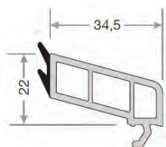
VETROCAMERA 23 • 24 MM • 25
